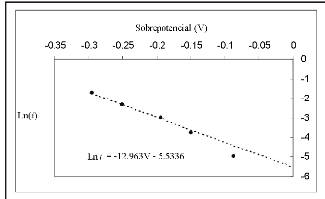
Figura 1. Característica de corriente-sobrepotencial
