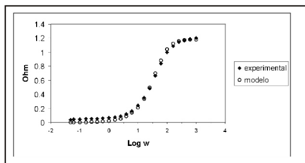
Figura 4. Comparación entre la impedancia calculada y experimental (5 Voltios rms, 0.05 - Hz, voltaje de operación 800 mV).
