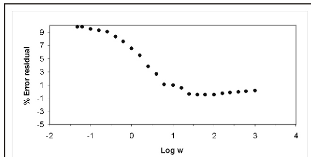
Figura 5. Análisis residuales (5 Voltios rms, 0.05-1000 Hz, 800 mV)
