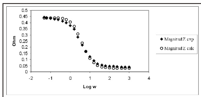
Figura 2. Curva experimental y calculada para la impedancia. Sobrepotencial directo 90 mV.
