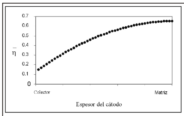
Figura 6. Sobrepotencial directo en el cátodo (150 mV en el colector)
